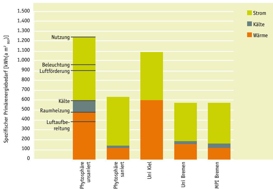
Abb. 1 Kennwerte des spezifischen Energieverbrauchs von Laborgebäuden [Jülich 2008]. Es handelt sich hier um Gebäude, die einen Labor- und einen Bürobereich besitzen.
