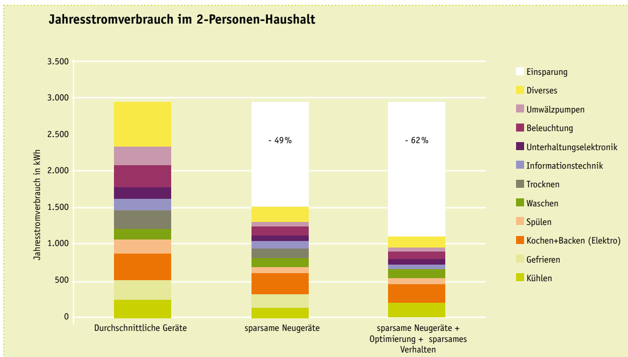
Abb. 3 Stromverbrauch im 2-Personen-Haushalt, abhängig von der energietechnischen Qualität der eingesetzten Geräte [Grafik nach Energiesparen im Haushalt, 2011]
