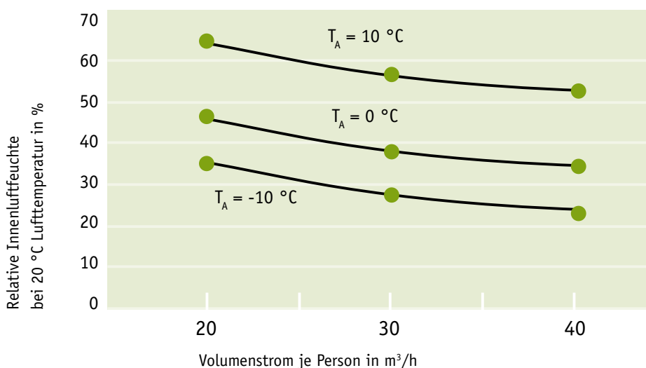
Abb. 5 Raumluftfeuchte bei verschiedenen Außenlufttemperaturen als Funktion des Frischluft-Volumenstroms je Person (Feuchtequellstärke je Person 90 g/h) [Werner 2004]
