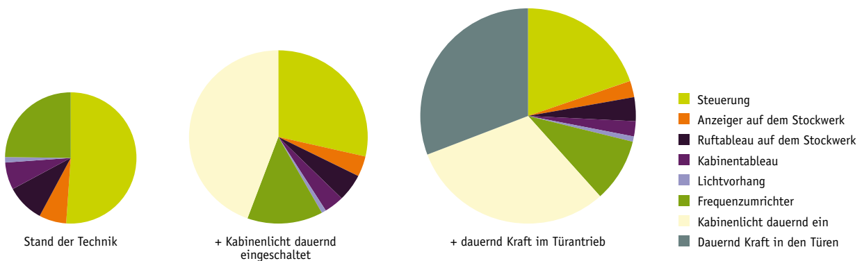
Abb. 4 Unterschiede im Stand-by-Betrieb von Aufzugsanlagen zwischen 40 Watt bei guter technischer Lösung (Stand der Technik) und 150 W bei technisch suboptimaler Ausführung [Nipkow06]
