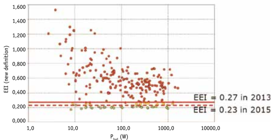
Abb. 7 Auswirkung der beschlossenen Anforderungen auf das Angebot an Heizungsumwälzpumpen (Quelle Europump/VDMA)
